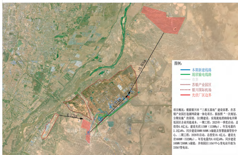
苏银产业园源网荷储项目示意图
